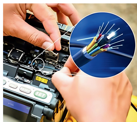
SPLICING FIBER OPTIC CABLE لحام كابل الفايبر
